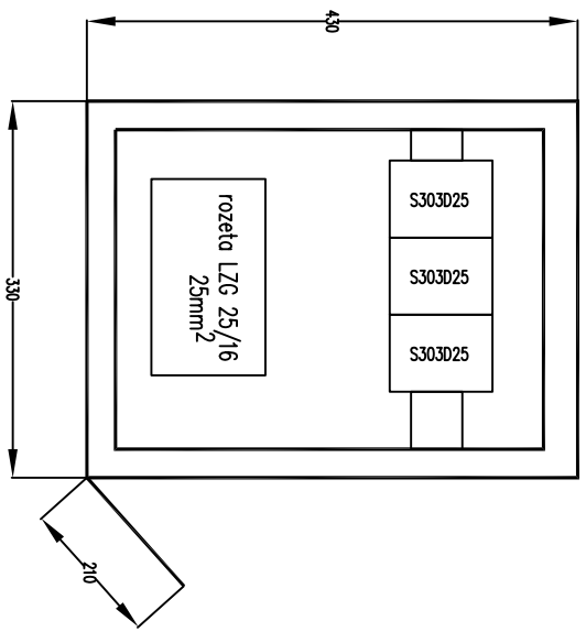
tablica wnękowa np. typu RWN 2x12 prod. LEGRAND
