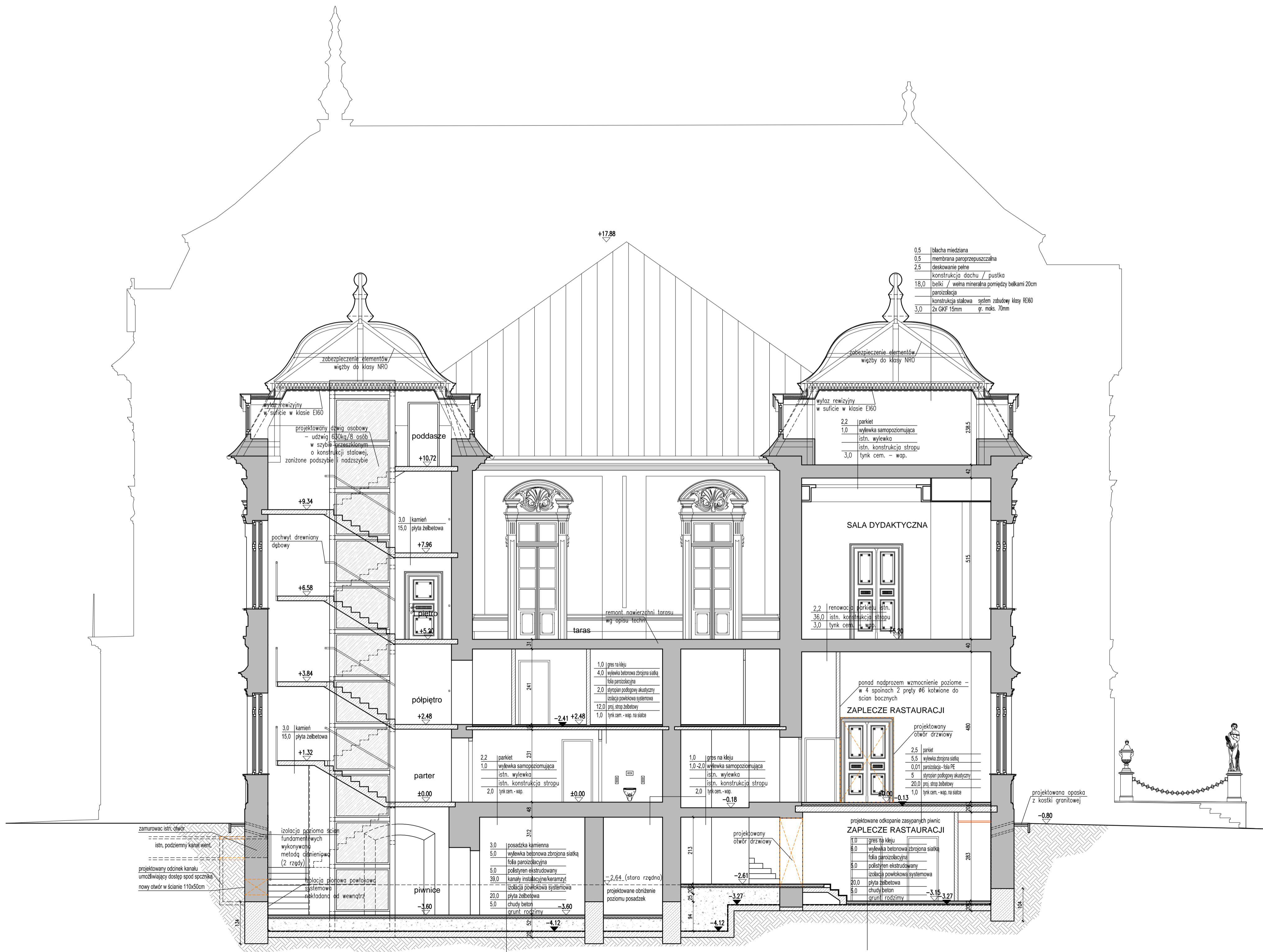
PRZEKRÓJ A - A
