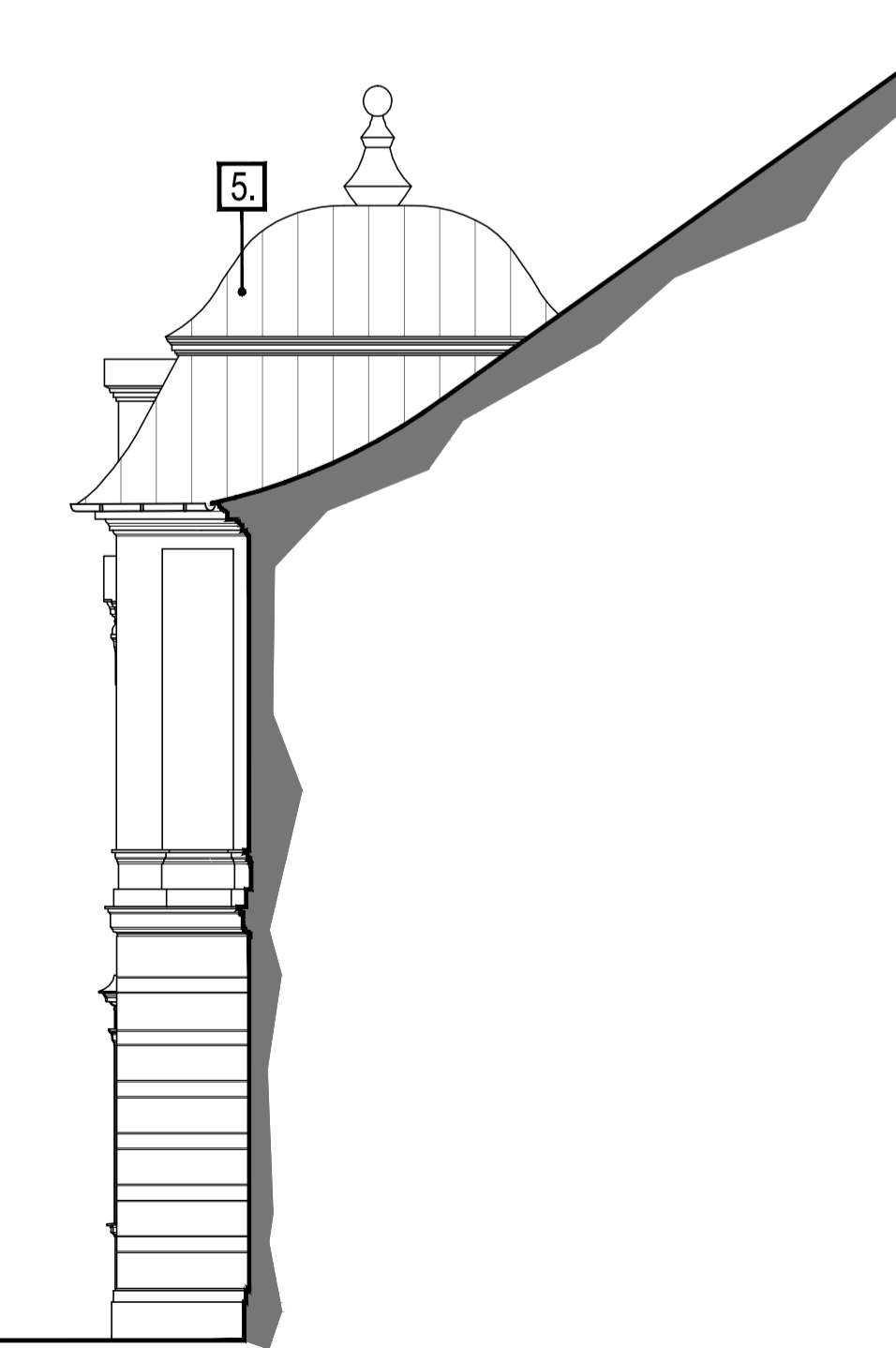
ELEWACJE BOCZNE ALKIERZA PÓŁNOCNO - ZACHODNIEGO
