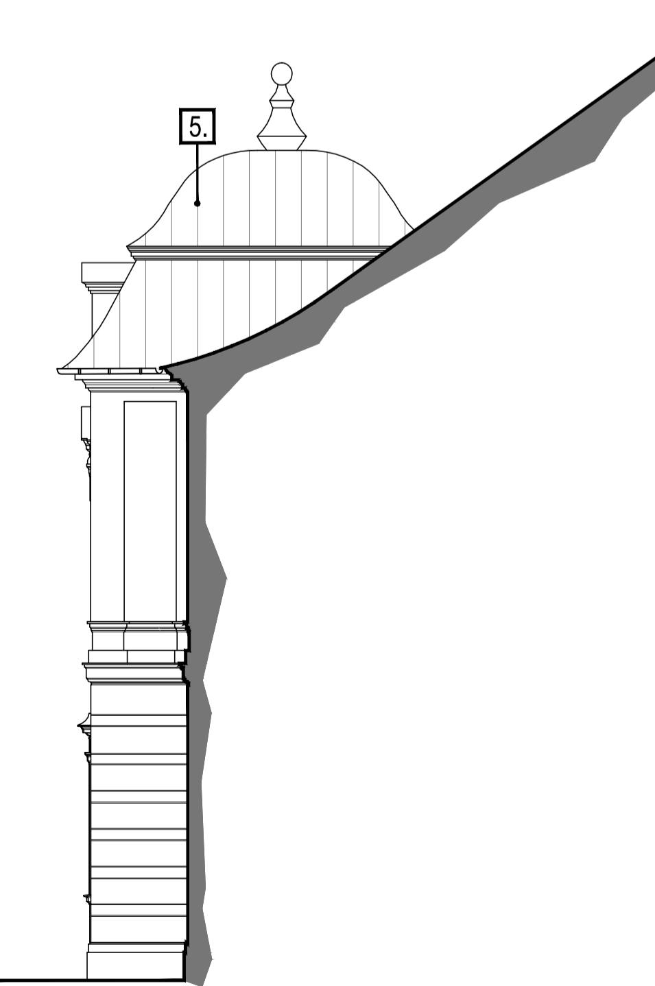
ELEWACJE BOCZNE ALKIERZA POŁUDNIOWO - WSCHODNIEGO
