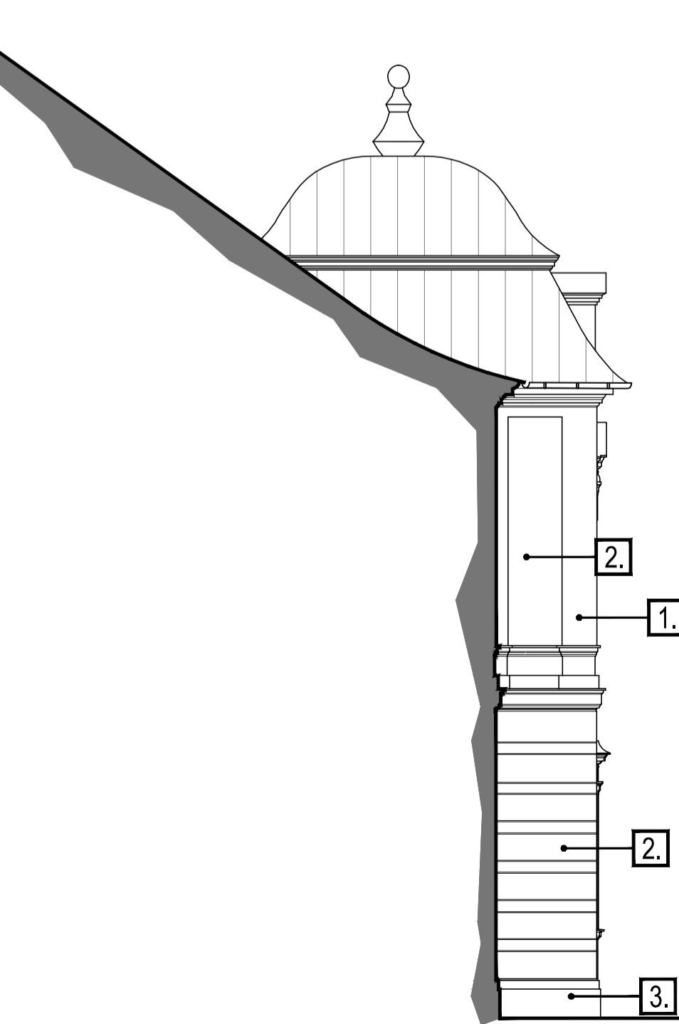
ELEWACJE BOCZNE ALKIERZA PÓŁNOCNO - WSCHODNIEGO
