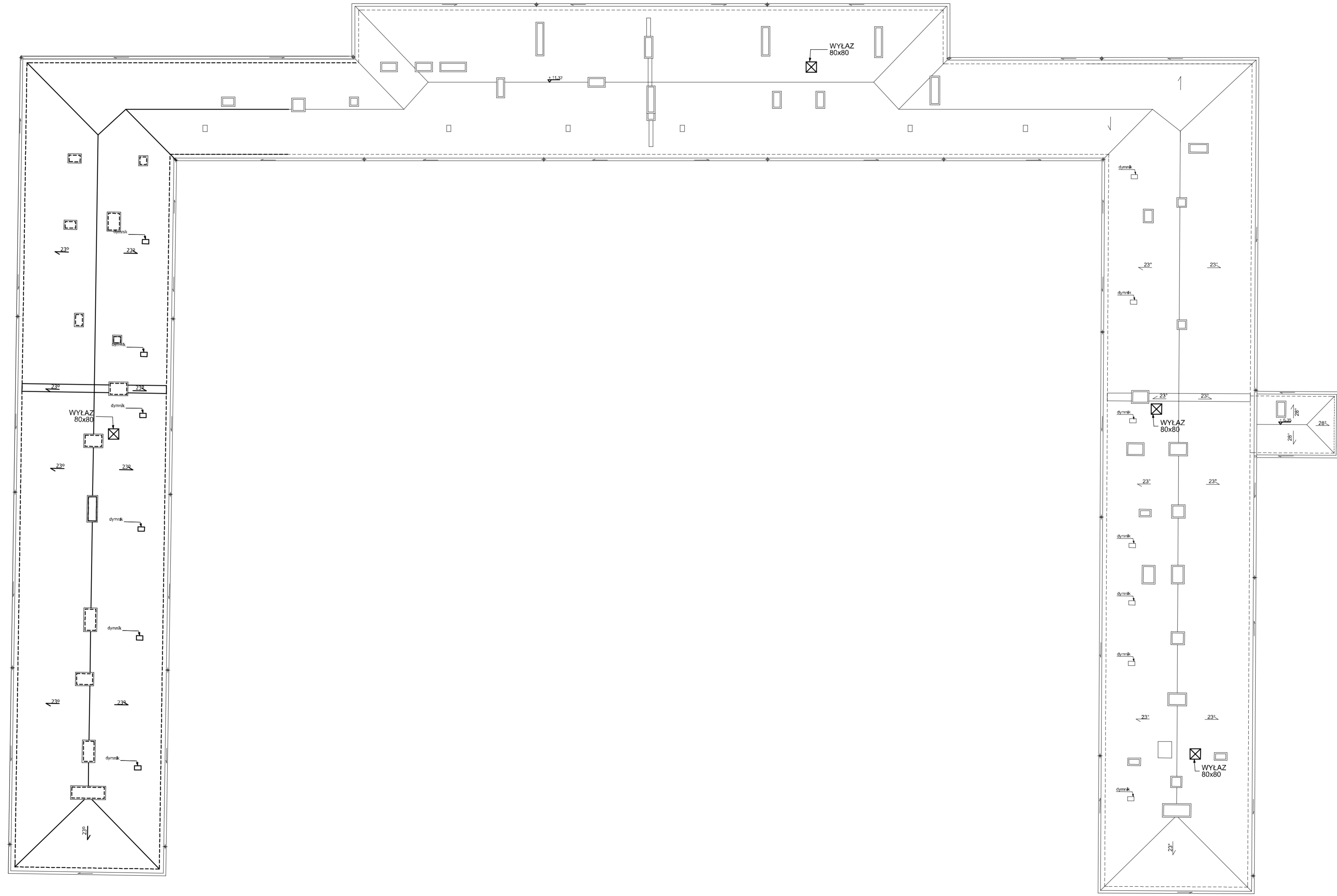
RZUT DACHU SKALA 1:200
